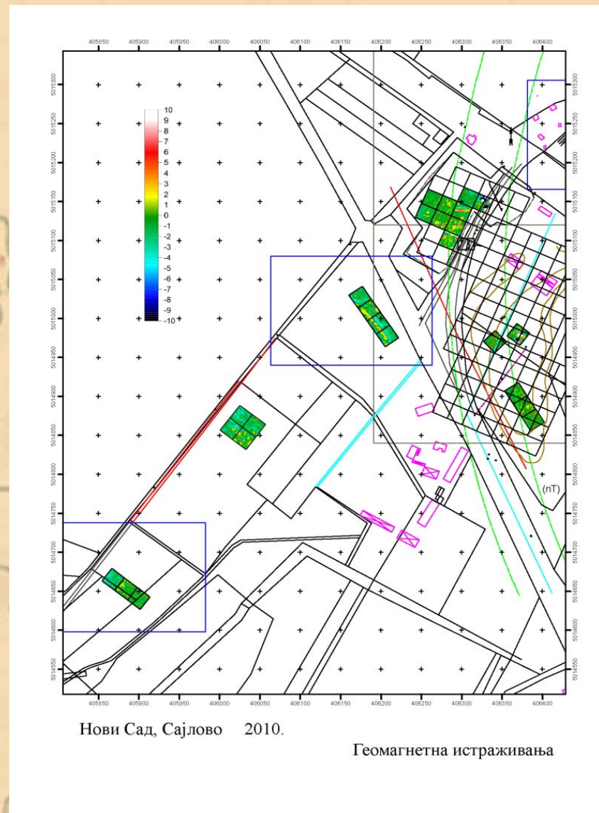
Резултати геомагнетних истраживања извршених на 10 000 m 2
